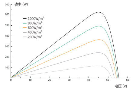
功率 - 电压曲线 (640W)
